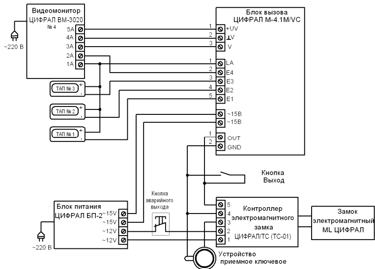
Рисунок Б.4 Схема подключения домофона ЦИФРАЛ М-4.1М/ВС
